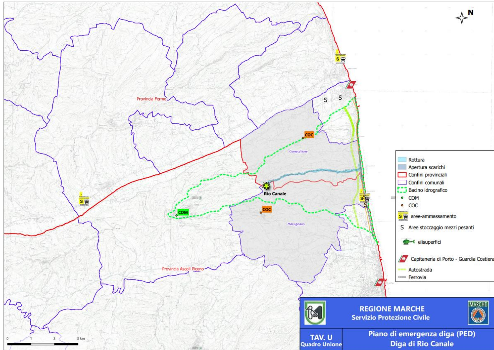
Piano di Emergenza Diga Diga di Rio Canale
